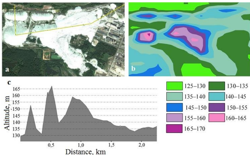
Рис. 2. Техногенный рельеф, образованный отвалами фосфогипса Гомельского химического завода: a – космический снимок; b – карта высот; c – гипсометрический профиль в пределах отвалов фосфогипса. [Fig. 2. Technogenic relief made by phosphogypsum dumps of the Gomel chemical plant: a – space image; b – altitude map; c – hypsometric profile.]
