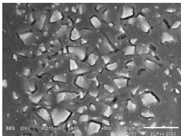
Рис. 1. РЭМ-изображения поверхности сульфокатионообменных мембран МК-40 при увеличении 500. Размер частиц ионообменной смолы < 20 мкм (а), 56–71 мкм (б)
