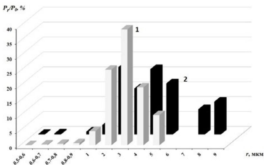
Рис. 3. Доли макропор P_r разного радиуса r от их общей площади P_0 на поверхности мембраны МК-40 с размером частиц ионообменной смолы < 20 мкм (1) и 56-71 мкм (2)
