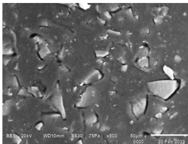
Рис. 1. РЭМ-изображения поверхности сульфокатионообменных мембран МК-40 при увеличении 500. Размер частиц ионообменной смолы < 20 мкм (а), 56–71 мкм (б)
