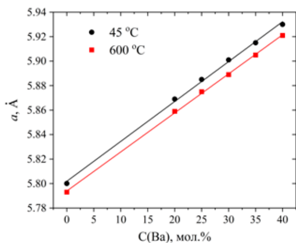
Рис. 2. Зависимость параметров решетки твердого раствора \text{Sr}_{0.925-x}\text{Ba}_x\text{Eu}_{0.075}\text{F}_{2.075} от содержания Ba
