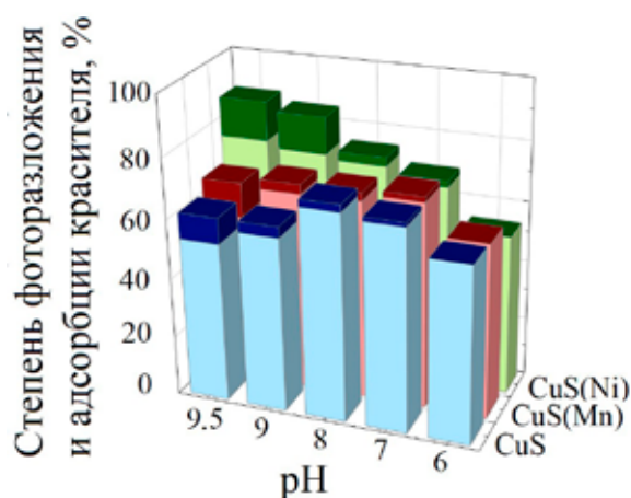
Рис. 10. Зависимость адсорбционной способности (нижняя часть) и фотокаталитической активности (верхняя часть) порошков-фотокатализаторов CuS(Mn) и CuS(Ni) от pH раствора красителя МС
