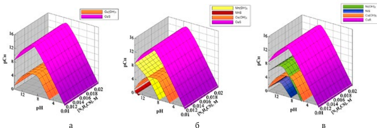
Рис. 2. Граничные условия образования труднорастворимых фаз CuS, MnS, NiS, Cu(OH) 2 , Mn(OH) 2 , Ni(OH) 2 в системах «CuCl 2 – CH 3 COONa – N 2 H 4 CS» (а), «CuCl 2 – MnCl 2 – CH 3 COONa – N 2 H 4 CS» (б) и «CuCl 2 – NiSO 4 – CH 3 COONa – N 2 H 4 CS» (в) в зависимости от pH среды и концентрации халькогенизатора. Расчеты проведены при [NaAc] = 2 М и T = 298 К
