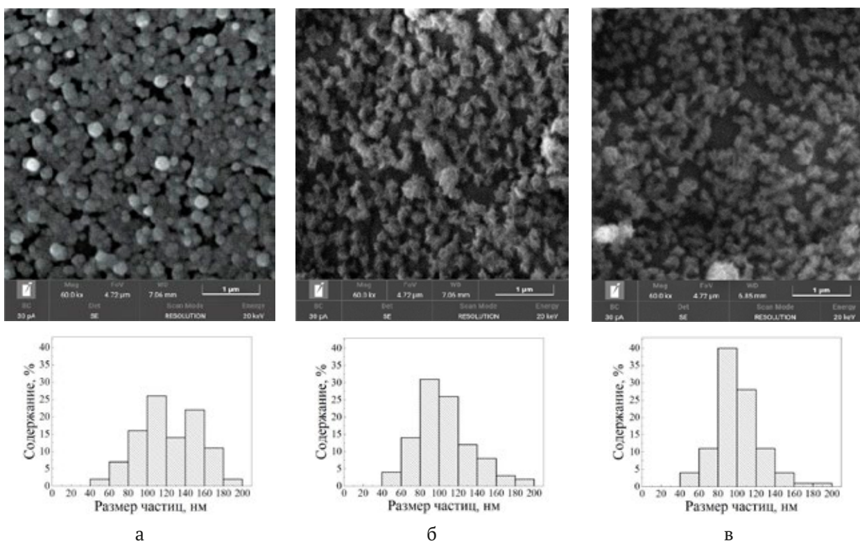
Рис. 3. Электронно-микроскопические изображения пленок нелегированного сульфида меди (а), а также CuS, легированного марганцем (б) и никелем (в), совместно с гистограммами распределения частиц по размерам
