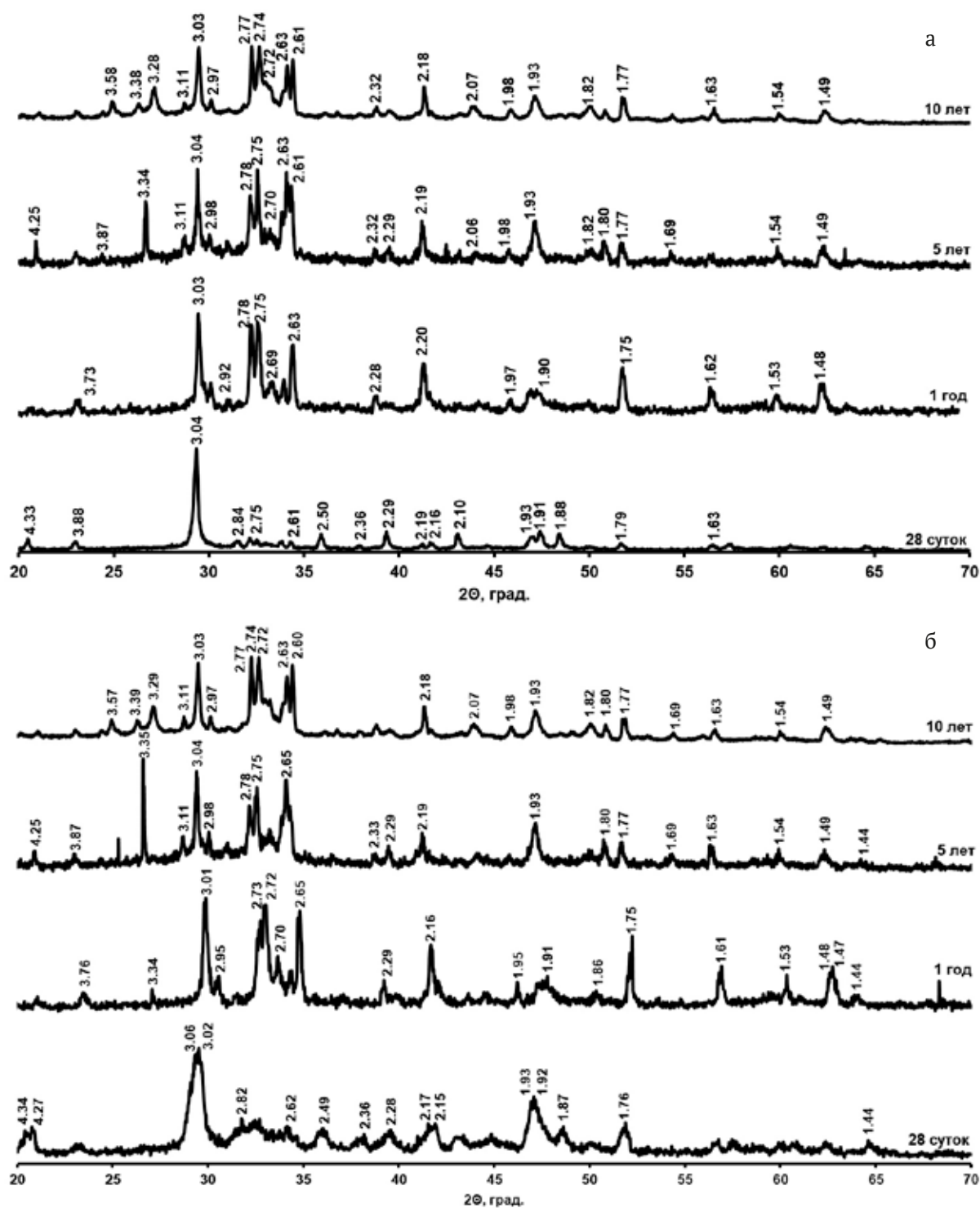
Рис. 1. Дифрактограммы наномодифицированных цементных систем: а) Ц – КНД; б) Ц – УНТ (\text{CaO})_x \cdot \text{SiO}_2 \cdot z\text{H}_2\text{O} ( d = 3.34; 3.05; 2.93; 2.80; 2.31; 1.83 ); \text{CaO} \cdot \text{SiO}_2 \cdot \text{H}_2\text{O} ( d = 4.24; 3.01; 2.78; 2.50; 2.23; 1.77 ); 2\text{CaO} \cdot \text{SiO}_2 \cdot \text{H}_2\text{O} ( d = 3.34; 3.01; 2.92; 2.25; 1.96; 1.81 ); 3\text{CaO} \cdot \text{SiO}_2 \cdot 2\text{H}_2\text{O} ( d = 3.33; 3.04; 2.92; 2.84; 1.88; 1.77 ); 3(2\text{CaO} \cdot \text{SiO}_2) \cdot \text{H}_2\text{O} ( d = 3.07; 2.97; 2.72; 2.62; 2.22; 1.74 ); 2\text{CaO} \cdot 3\text{SiO}_2 \cdot \text{H}_2\text{O} ( d = 4.24; 3.84; 3.36; 3.15; 2.85; 2.25 ); 3\text{CaO} \cdot 2\text{SiO}_2 \cdot 3\text{H}_2\text{O} ( d = 3.05; 2.74; 2.31; 2.21; 1.92; 1.68 ); 2\text{CaO} \cdot \text{SiO}_2 \cdot 0.5\text{H}_2\text{O} ( d = 2.99; 2.77; 2.67; 2.25; 1.80; 1.61 ); 6\text{CaO} \cdot 6\text{SiO}_2 \cdot 2\text{H}_2\text{O} ( d = 3.65; 3.23; 3.07; 2.83; 2.04; 1.95 ); \text{CaO} \cdot \text{Al}_2\text{O}_3 \cdot 8.5\text{H}_2\text{O} ( d = 3.57; 3.13; 2.75; 2.58; 2.34; 1.79 ); 4\text{CaO} \cdot \text{Al}_2\text{O}_3 \cdot 19\text{H}_2\text{O} ( d = 2.88; 2.78; 2.67; 2.35; 1.93; 1.82 ); 3\text{CaO} \cdot \text{Al}_2\text{O}_3 \cdot \text{SiO}_2 \cdot 4\text{H}_2\text{O} ( d = 3.07; 2.74; 2.24; 1.99; 1.70; 1.64 ); \text{CaO} \cdot \text{Al}_2\text{O}_3 \cdot 2\text{SiO}_2 \cdot 4\text{H}_2\text{O} ( d = 3.34; 3.19; 2.74; 2.70; 2.66; 1.81 ); 3\text{CaO} \cdot \text{Fe}_2\text{O}_3 \cdot \text{CaSO}_4 \cdot 16\text{H}_2\text{O} ( d = 3.40; 2.93; 2.55 ); 3\text{CaO} \cdot \text{Al}_2\text{O}_3 \cdot 3\text{CaSO}_4 \cdot 32\text{H}_2\text{O} ( d = 4.90; 3.02; 2.79; 1.62; 1.54; 1.50 ); \text{Ca}(\text{OH})_2 ( d = 3.11; 2.63; 1.93; 1.79; 1.69; 1.49 ) [19]
