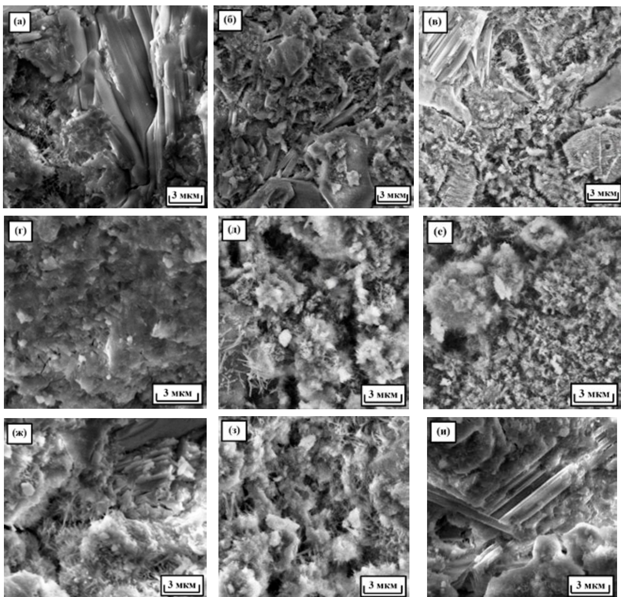
Рис. 3. Микрофотографии исследуемых цементных систем: Ц – В (а, б, в); Ц – КНД (г, д, е); Ц – УНТ (ж, з, и) при различной продолжительности твердения (28 суток – а, г, ж; 5 лет – б, д, з; 10 лет – в, е, и)
