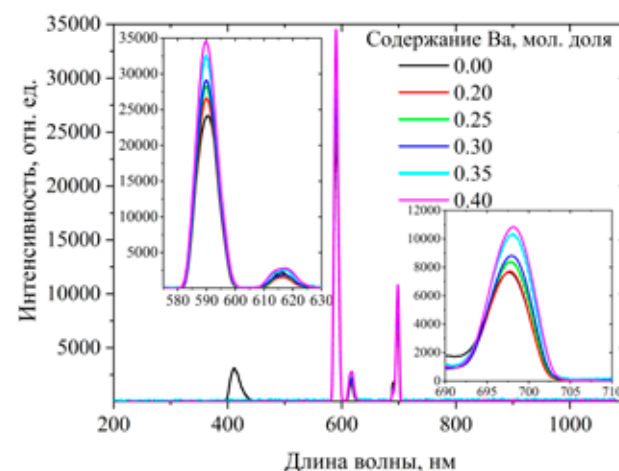
Рис. 3. Спектры рентгенолюминесценции твердого раствора \text{Sr}_{0.925-x}\text{Ba}_x\text{Eu}_{0.075}\text{F}_{2.075}
