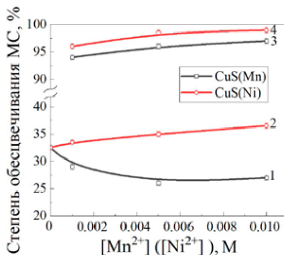
Рис. 9. Зависимость степени обесцвечивания красителя МС в присутствии пленок (1, 2) и порошков (3, 4) CuS(Mn) (1, 3) CuS(Ni) (2, 4) от концентрации соли марганца (никеля) в реакционной смеси
