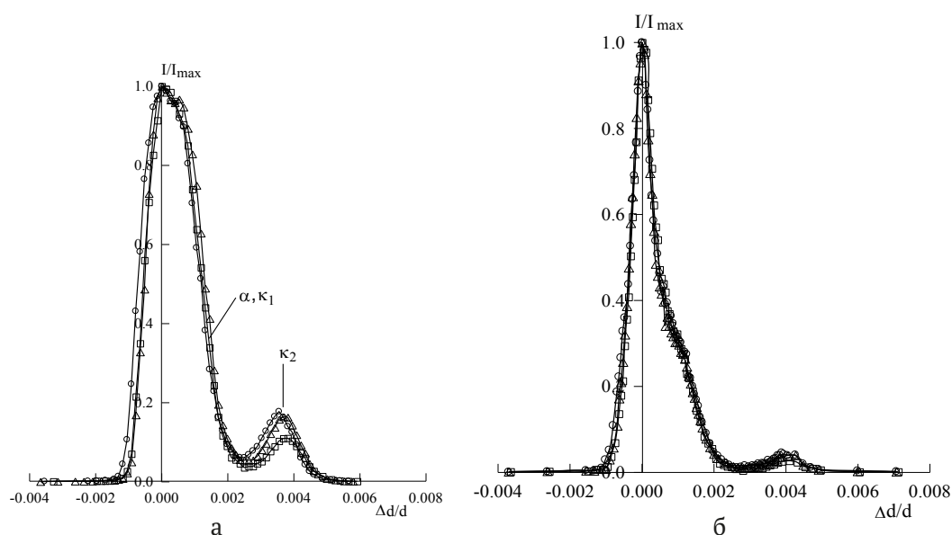
Рис. 5. \theta/2\theta -кривые протоннообменных слоев на ниобате лития после ПО 175 °С, 6 ч и отжига 370 °С, 2 ч: (○) ПО в ОБК, (△) ПО в НБК, (□) ПО в ВБК. Отражение от плоскостей: а – (110), б – (220)
