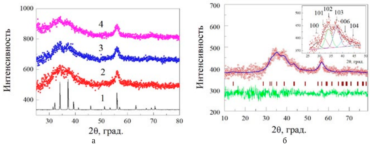
Рис. 6. Экспериментальные рентгенограммы пленок CuS (2), CuS(Mn) (3), CuS(Ni) (4) сдвинуты по оси ординат для наглядности. Расчетная рентгенограмма эталонного CuS (1) гексагональной структуры ковеллина (пр. гр. P6_3/mmc ) (а). Экспериментальная рентгенограмма (красные кружки), а также расчетная (синяя линия) и разностная (зеленая линия) кривые для CuS(Mn). Угловые положения брэггльских рефлексов изображены штрихами (б). На вставке показано разложение профиля на отдельные пики
