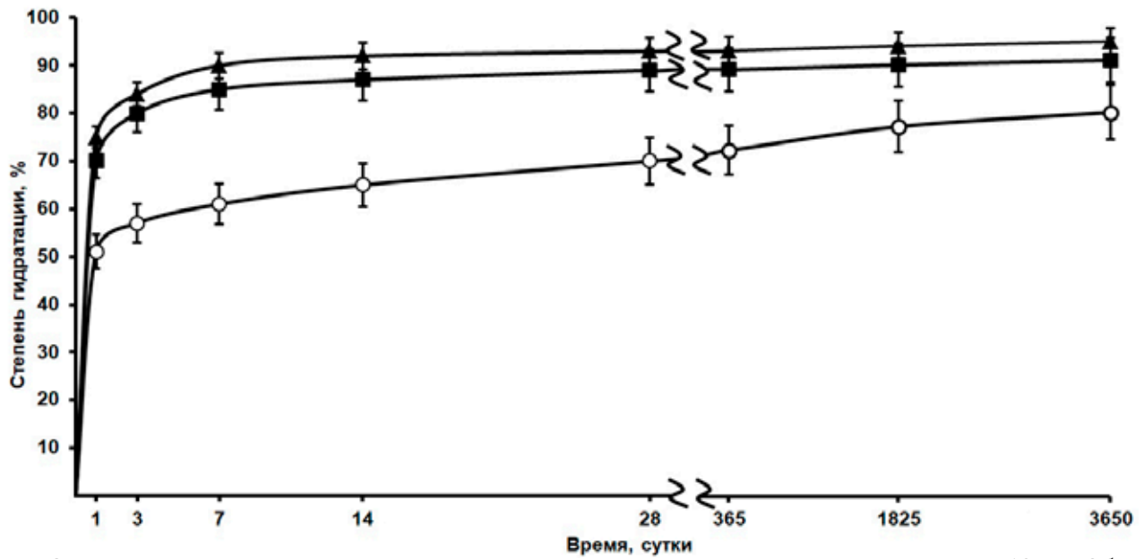
Рис. 2. Кинетика гидратации цементных систем при продолжительности их твердения до 10 лет. Обозначено: ○ – Ц – В; ▲ – Ц – КНД; ■ – Ц – УНТ
