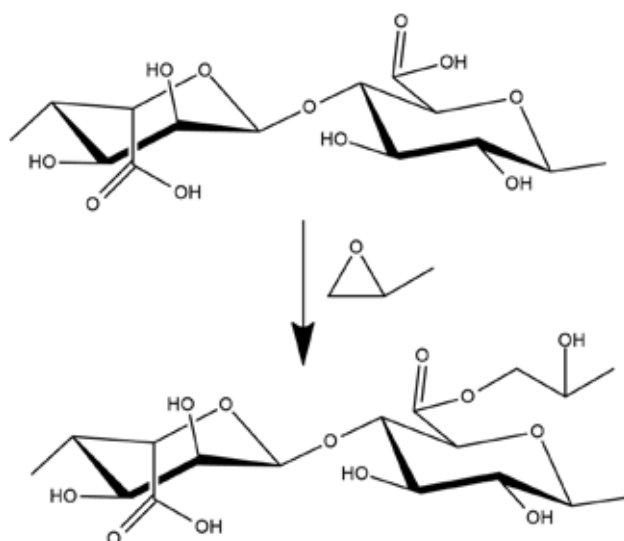
Рис. 1. Схема процесса синтеза пропиленгликоль альгината
