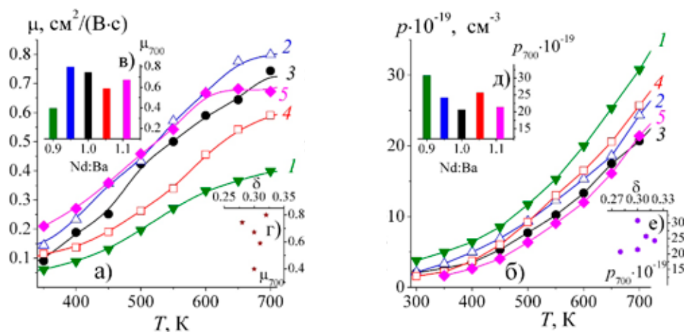
Рис. 5. Зависимости взвешенной подвижности (а, в, г) и концентрации носителей заряда (б, д, е) от температуры (а, б) и состава (в–е) керамики N090B (1), N095B (2), NB (3), NB095 (4), NB090 (5)
