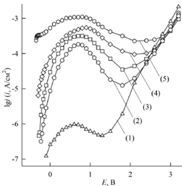
Рис. 1. Анодные потенциостатические кривые MnSi-электрода в растворах 0.5 М H_2SO_4 (1) и 0.5 М H_2SO_4 + (x) М NaF, где x = 0.0025 (2); 0.005 (3); 0.01 (4), 0.05 (5)
