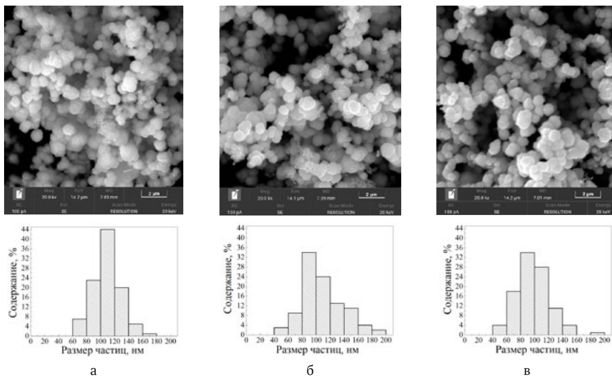
Рис. 4. Электронно-микроскопические изображения порошков нелегированного сульфида меди (а), а также CuS, легированного марганцем (б) и никелем (в), совместно с гистограммами распределения частиц по размерам
