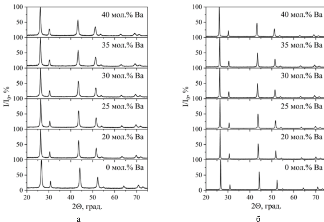
Рис. 1. Рентгенограммы синтезированных образцов твердых растворов \text{Sr}_{0.925-x}\text{Ba}_x\text{Eu}_{0.075}\text{F}_{2.075} : а – после сушки на воздухе при температуре 45 °С, б – после термообработки при температуре 600 °С
