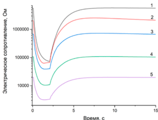
Рис. 4. Электрическое сопротивление сенсора WO_3 -Pd при различных концентрациях сероводорода на протяжении одного измерительного цикла. 1 – синтетический воздух, 2 – 5 ppm H_2S , 3 – 10 ppm H_2S , 4 – 20 ppm H_2S , 5 – 50 ppm H_2S
