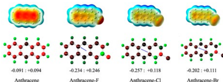
Рис. 6. Карта распределения электростатического потенциала и распределение заряда антрацена и его структур, легированных галогенами
