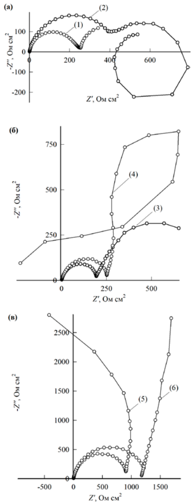
Рис. 6. Спектры импеданса MnSi-электрода в растворе 0.5 М H 2 SO 4 + 0.05 М NaF при E, В: -0.32 (1); 0 (2); 0.9 (3); 1.1 (4); 1.8 (5); 2.6 (6)
