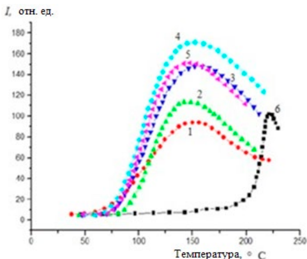
Рис. 1. Кривые термического высвечивания образцов \text{PbCd}_{2-x}\text{B}_6\text{O}_{12} : x\text{Cu}^{2+} с x = 0.03 (1), 0.05 (2), 0.07 (3), 0.06 (4), 0.08 (5); LiF – (6) при возбуждении УФ в течение 5 мин
