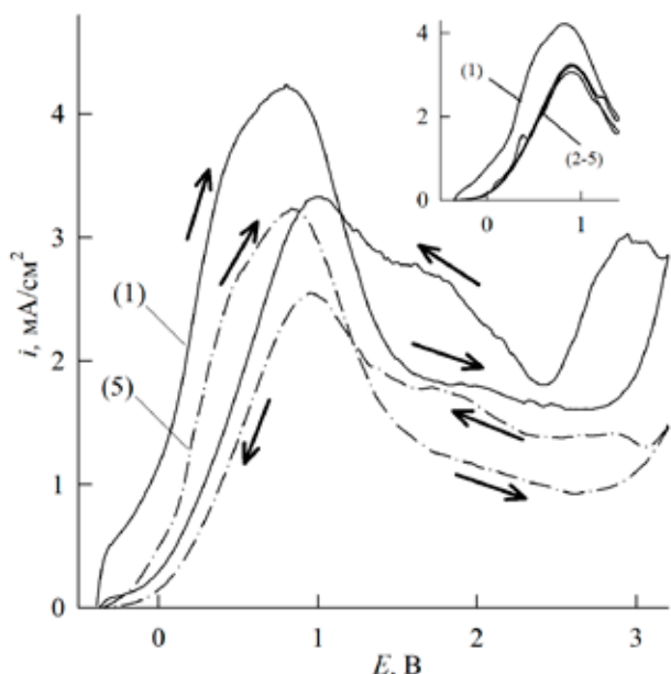
Рис. 4. Циклические вольтамперные кривые MnSi-электрода в растворе 0.5 \text{ M H}_2\text{SO}_4 + 0.05 \text{ M NaF} . Номер – цикл поляризации. В верхнем правом углу – 5 циклов поляризации при потенциале реверса E_{\text{реверс}} = 1.4 В
