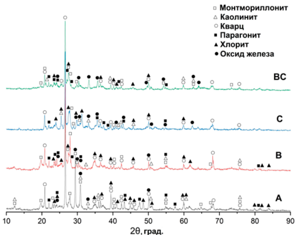
Рис. 4. Дифрактограммы образцов: А, В, С, ВС (снизу-вверх)
