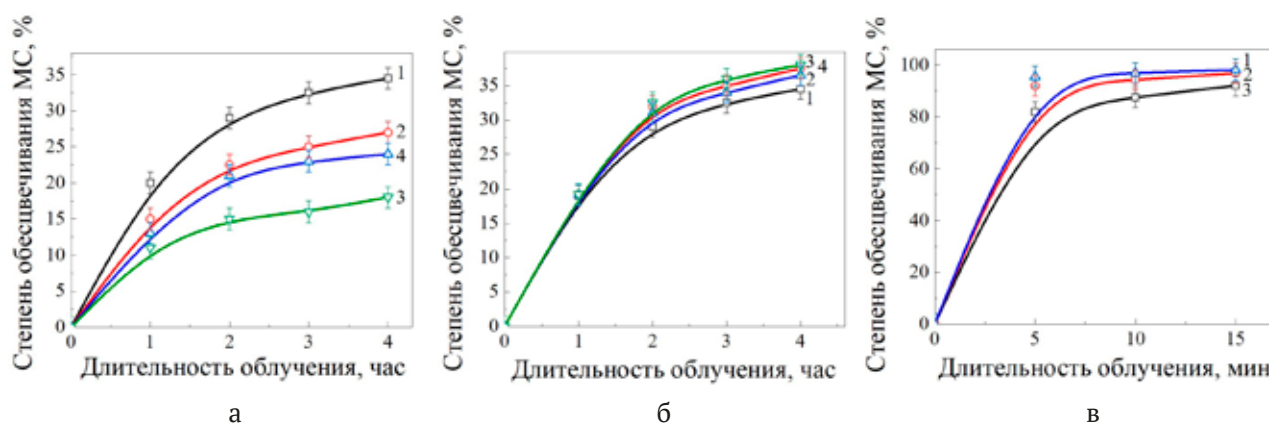
Рис. 8. Зависимость степени обесцвечивания МС от длительности облучения светом видимого диапазона в присутствии пленок-катализаторов CuS(Mn) (а) и CuS(Ni) (б), полученных из реакционных смесей, содержащих 0 (1), 0.001 (2), 0.005 (3), 0.01 (4) М соли MnCl_2 или NiSO_4 соответственно, а также порошковых-катализаторов CuS(Ni) (1), CuS(Mn) (2), полученных из реакционных смесей, содержащих 0.005 М соли никеля (марганца), а также нелегированного CuS (3) (в)
