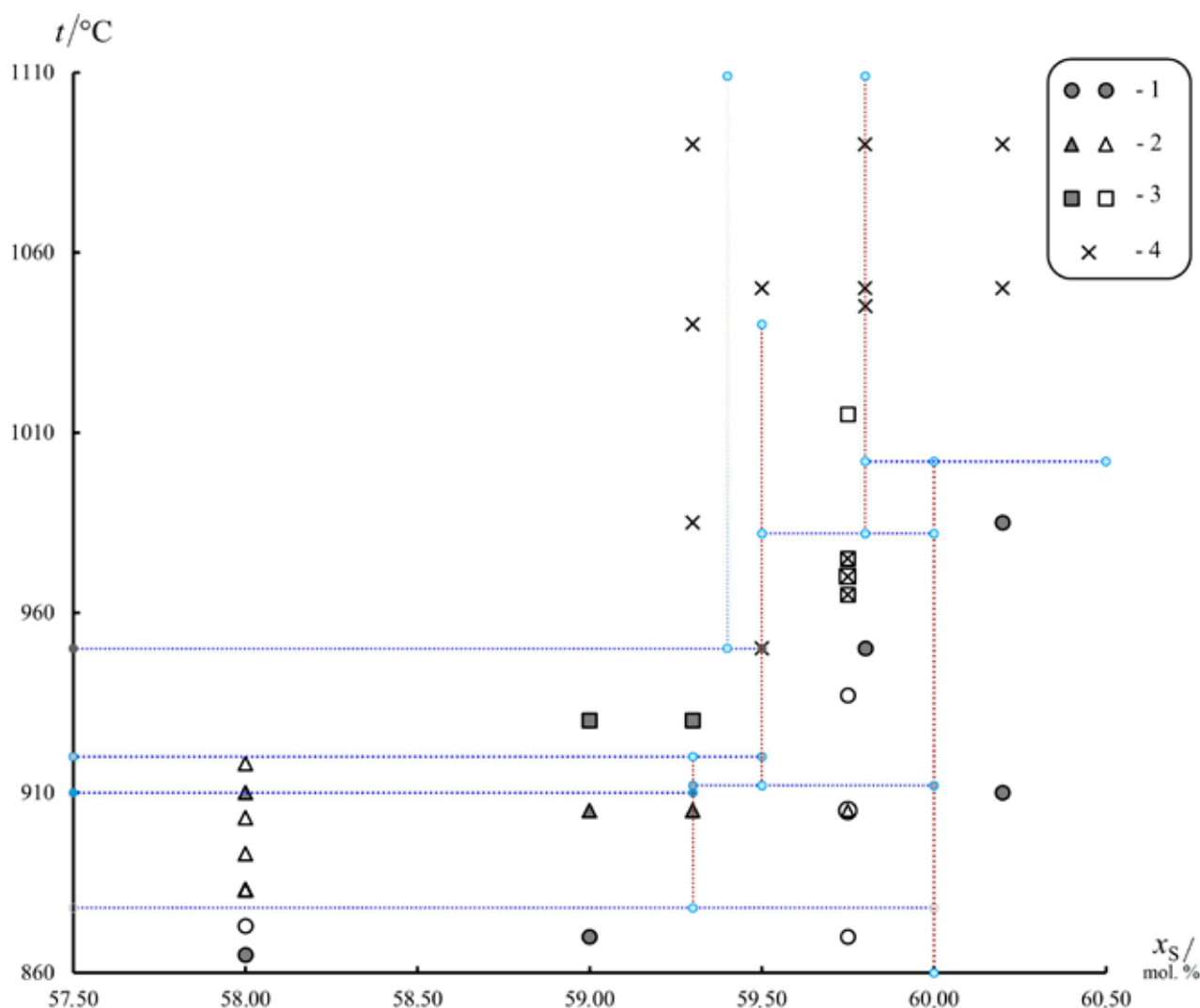
Рис. 2. Выявленные в ходе рентгеновского порошкового анализа составы образцов системы Ga – S, поставленные в соответствие T - x -координатам фазовой диаграммы. Обозначения. Отожженные и закаленные сплавы обозначены как темные, с серой заливкой фигурки – кружочки, треугольники, квадраты, крестики; образцы, исследованные in situ при высоких температурах в «синхротронном» эксперименте – светлые фигурки без заливки. Цифровые обозначения: 1 – \alpha' - \text{Ga}_2\text{S}_3 (+ следы GaS для составов с x_S < 60.0 мол. %), 2 – \gamma - \text{Ga}_{2+\delta}\text{S}_3 (+ следы GaS для температур меньше 910 °C), 3 – \beta - \text{Ga}_2\text{S}_3 , 4 – \alpha - \text{Ga}_2\text{S}_3 . Пунктирными линиями нанесены горизонтали, полученные по результатам ДТА, а также составы вероятных фаз (вертикальные пунктирные линии)
