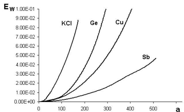
Рис. 2. Энергетические спектры тепловых флуктуаций в фазе предплавления KCl, Ge, Cu, Sb в стационарном режиме
