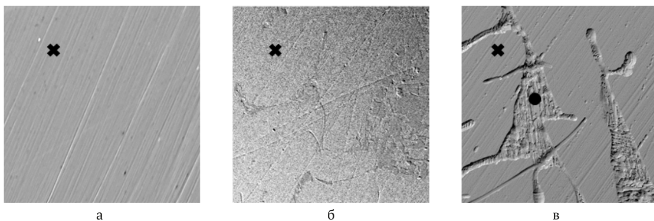
Рис. 2. Микрофотографии поверхности MnSi ( \times 400 ) до (а) и после травления в 0.5 М \text{H}_2\text{SO}_4 (б) и 0.5 М \text{H}_2\text{SO}_4 + 0.05 М NaF (в) при E = 3.2 В
