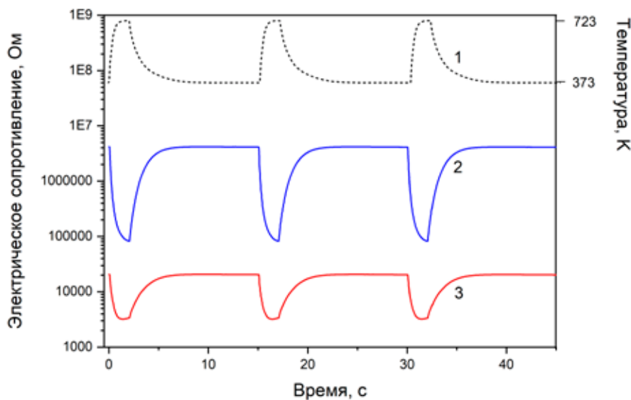
Рис. 3. Температура (кривая 1) и электрическое сопротивление сенсора \text{WO}_3 -Pd в 50 ppm угарного газа (кривая 2) и в 50 ppm сероводорода (кривая 3) в нестационарном температурном режиме на протяжении трех циклов измерений
