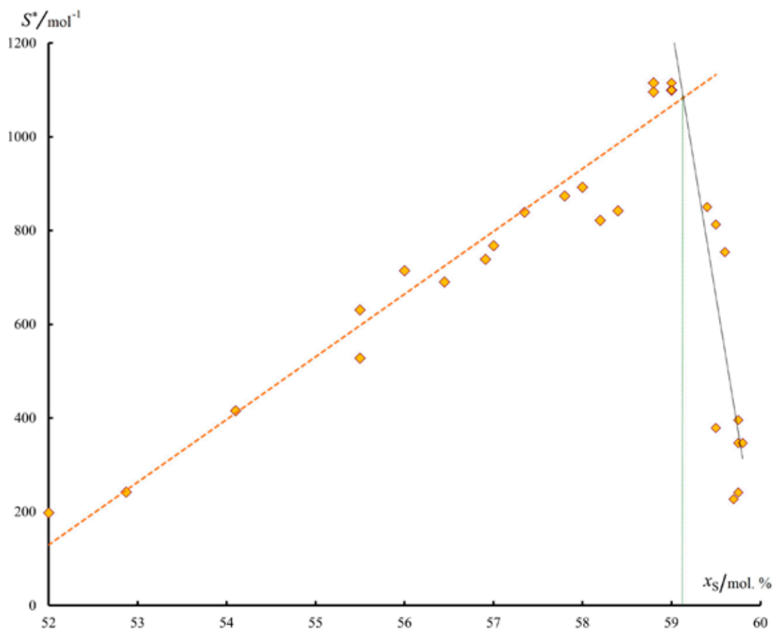
Рис. 3. Зависимость величины приведенной площади пиков на дифференциальных термо-граммах нагревания от составов сплавов для эндоэффекта, наблюдаемого при T \approx 878 °С
