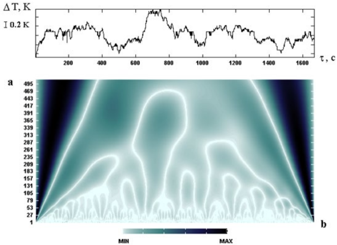
Рис. 1. Кривая ДТА и вейвлет-преобразование флуктуационного процесса предплавления Cu ( T^* = 1221.8 K)
