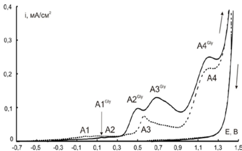
Рис. 1. Циклические вольтамперограммы, полученные на золотом электроде в фоновом растворе (пунктир) и с добавкой 0.03М глицина; v = 0.10 В/с [10]
