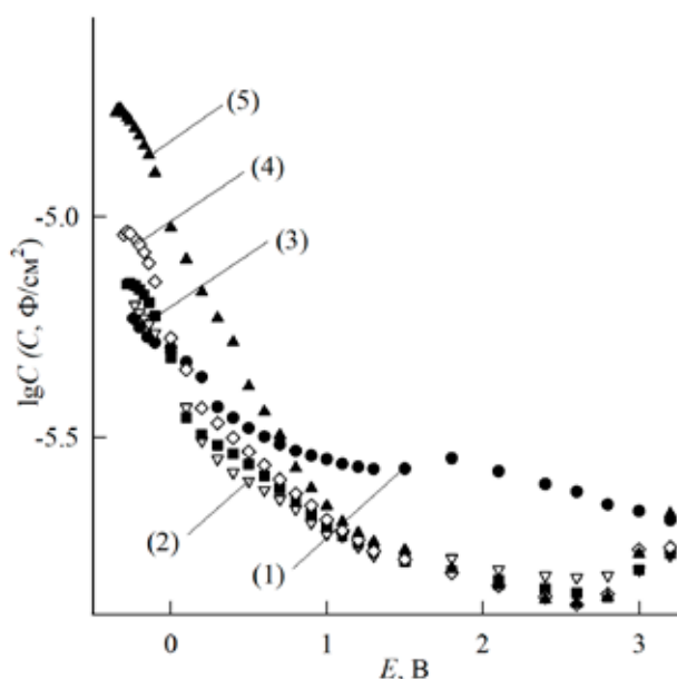
Рис. 5. Зависимость логарифма дифференциальной емкости от потенциала MnSi-электрода в растворах 0.5 \text{ M H}_2\text{SO}_4 (1) и 0.5 \text{ M H}_2\text{SO}_4 + (x) \text{ M NaF} , где x = 0.0025 (2); 0.005 (3); 0.01 (4), 0.05 (5)
