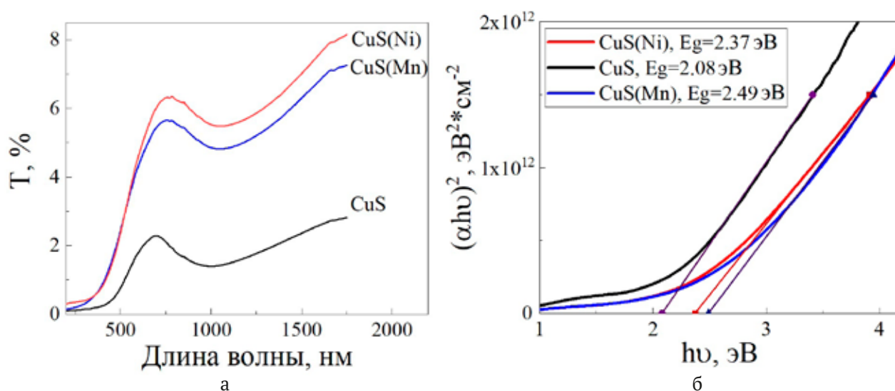
Рис. 7. Спектры светопропускания пленок CuS, CuS(Ni), CuS(Mn) (а); результаты графического определения ширины запрещенной зоны пленок (б)
