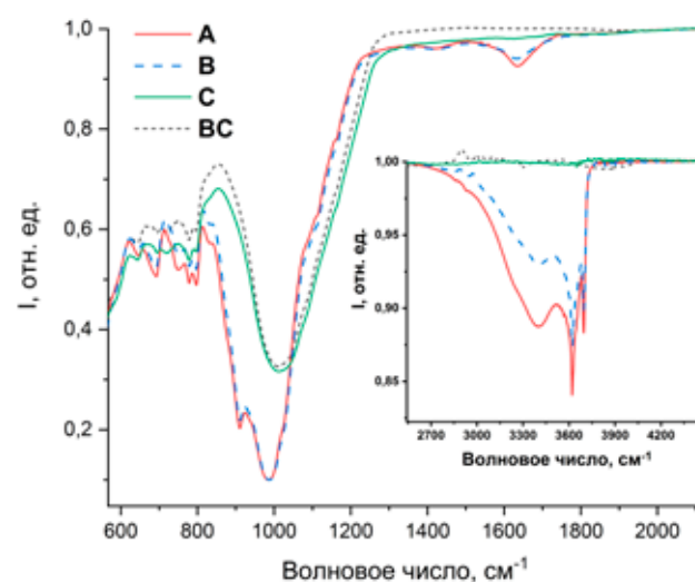
Рис. 3. ИК-спектры партий образцов: A , B , C , BC
