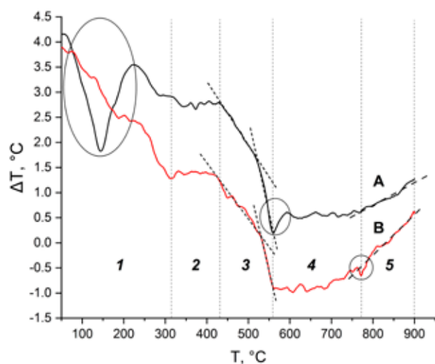
Рис. 2. Термограммы A - и B -проб
