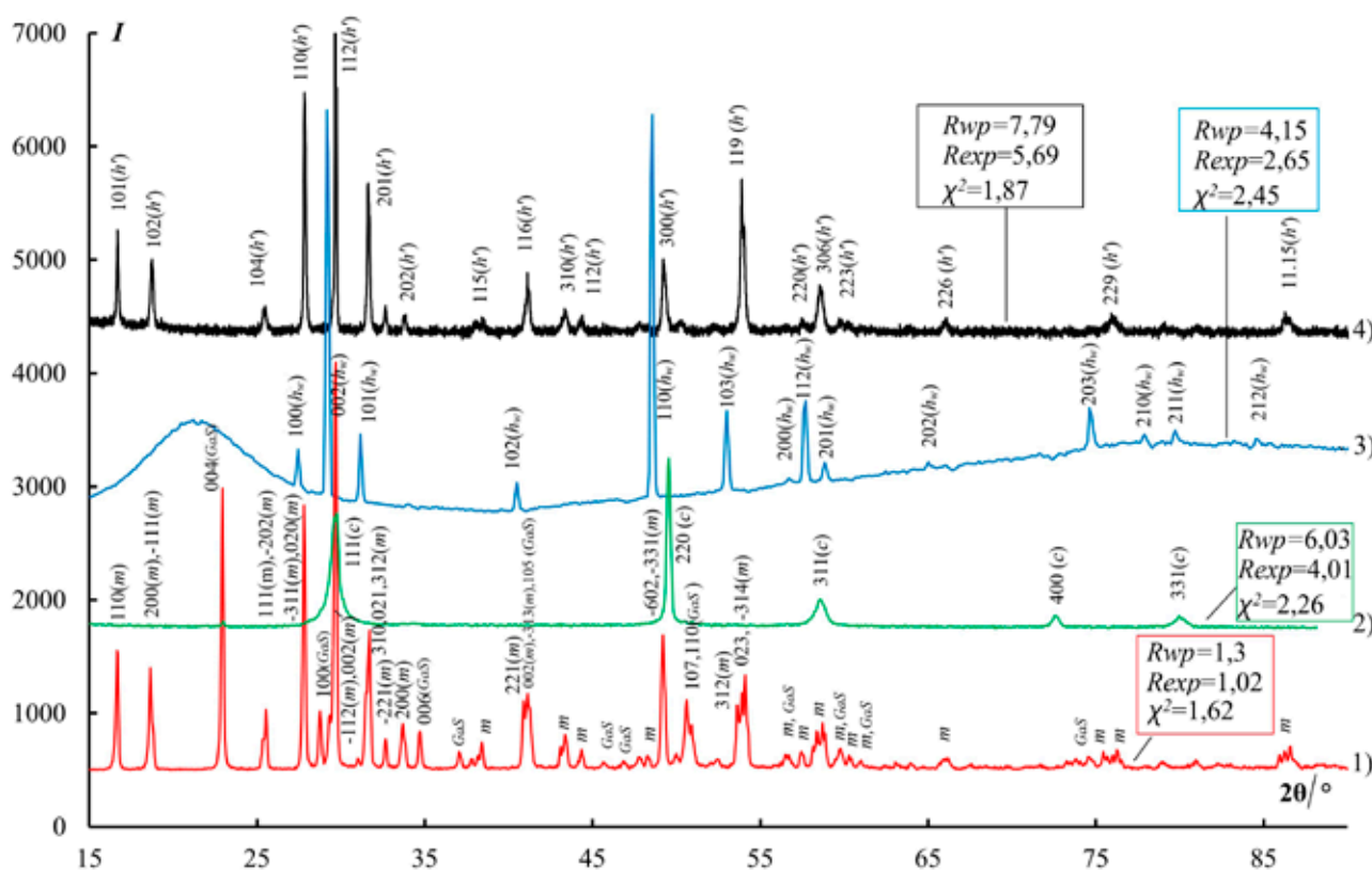
Рис. 1. Дифрактограммы для образцов системы Ga – S различных составов, полученные в разных условиях и идентифицируемые как: 1 – \alpha' - \text{Ga}_2\text{S}_3 ( m ) с примесью GaS; 2 – \gamma - \text{Ga}_{2+\delta}\text{S}_3 ( c ); 3 – \beta - \text{Ga}_2\text{S}_3 ( h_w ); 4 – \alpha - \text{Ga}_2\text{S}_3 ( h' ); в скобках указаны обозначения рефлексов для данной фазы. Кривые 1, 2, 4 соответствуют образцам, полученным в ходе отжигово-закалочных экспериментов; кривая 3 соответствует данным in-situ исследования с использованием синхротронного рентгеновского излучения с пересчетом результатов на «медное» излучение
