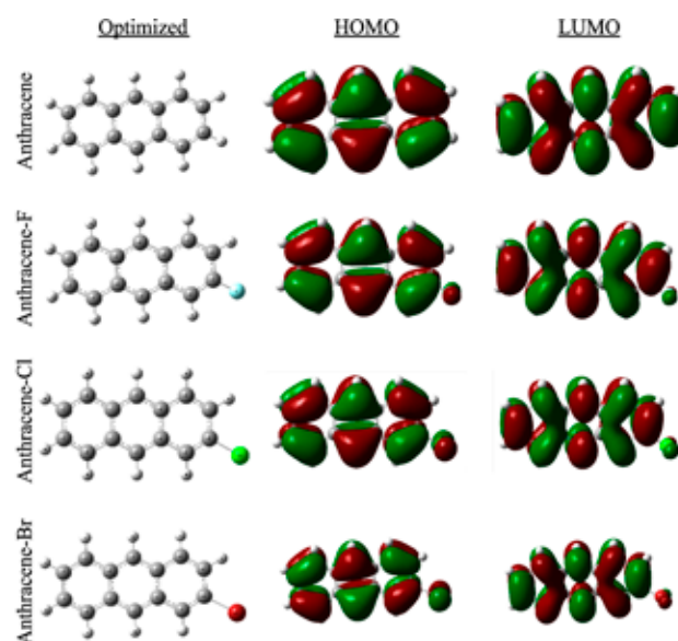
Рис. 1. Оптимизированные структуры и молекулярные орбитали антрацена и его структур, легированных галогенами
