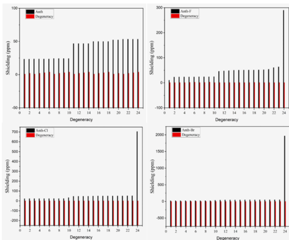
Рис. 5. ЯМР антрацена и его галогенсодержащих производных
