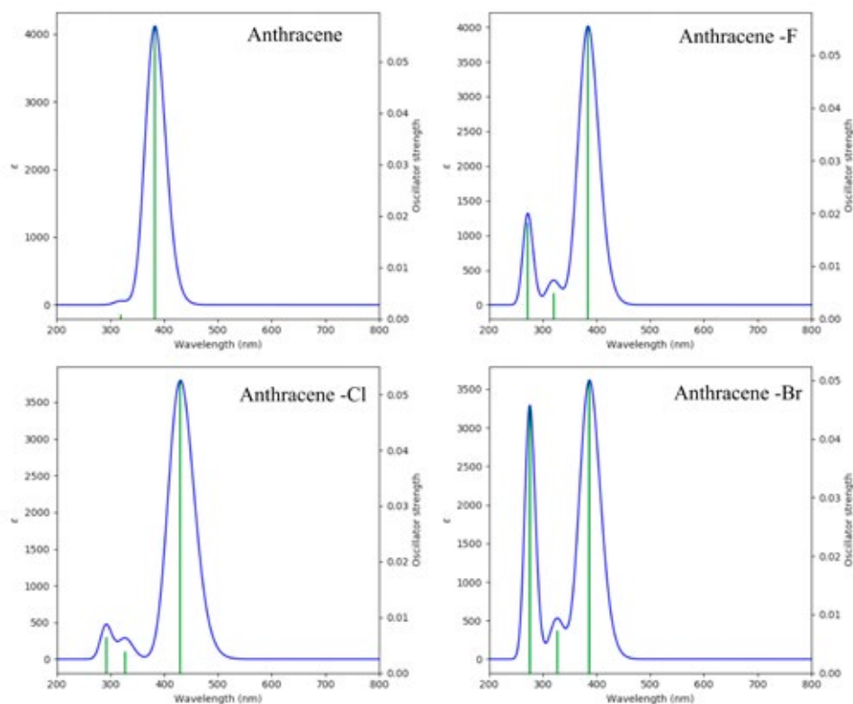
Рис. 3. Спектры поглощения излучения в видимом диапазоне для антрацена и его галогенсодержащих производных
