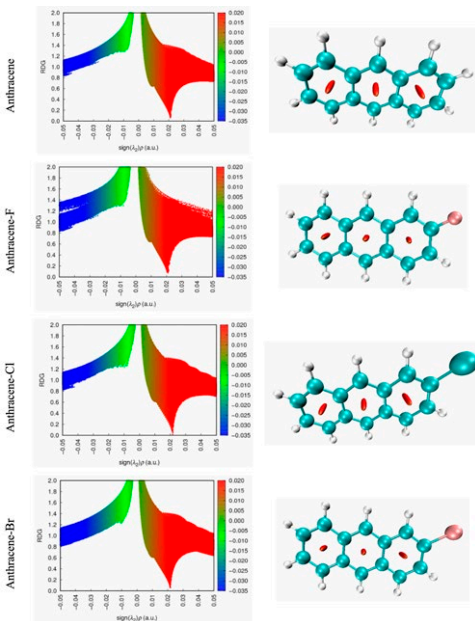
Рис. 7. Анализ RDG исследуемых соединений – слабые и сильные взаимодействия
