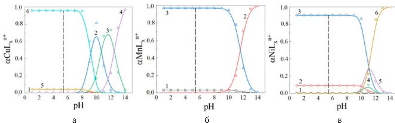
Рис. 1. Диаграммы ионных равновесий в системах (а) « CuCl_2 - CH_3COONa - N_2H_4CS »: CuOH^+(1), Cu(OH)_2(2), Cu(OH)_3^-(3), Cu(OH)_4^{2-}(4), CuCH_3COO^+(5), Cu(CH_3COO)_2(6) ; (б) « MnCl_2 - CH_3COONa - N_2H_4CS »: Mn^{2+}(1), MnOH^+(2), MnCH_3COO^+(3) ; (в) « NiSO_4 - CH_3COONa - N_2H_4CS »: Ni^{2+}(1), NiCH_3COO^+(2), Ni(CH_3COO)_2(3), NiOH^+(4), Ni(OH)_2(5), Ni(OH)_3^-(6)
