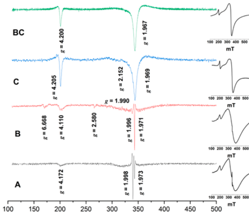
Рис. 5. ЭПР-спектры образцов: А, В, С, ВС (снизу-вверх)
