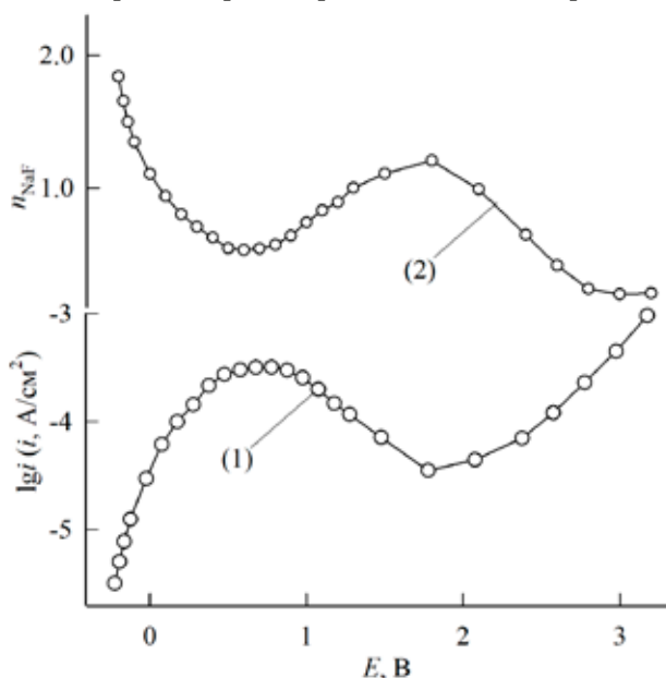
Рис. 3. Графики зависимостей электрохимических величин от потенциала MnSi -электрода: (1) Анодная потенциостатическая кривая в 0.5 М H_2SO_4 + 0.0025 М NaF ; (2) Зависимость n_{NaF} от потенциала в растворах 0.5 М H_2SO_4 + (0.0025–0.05) М NaF
