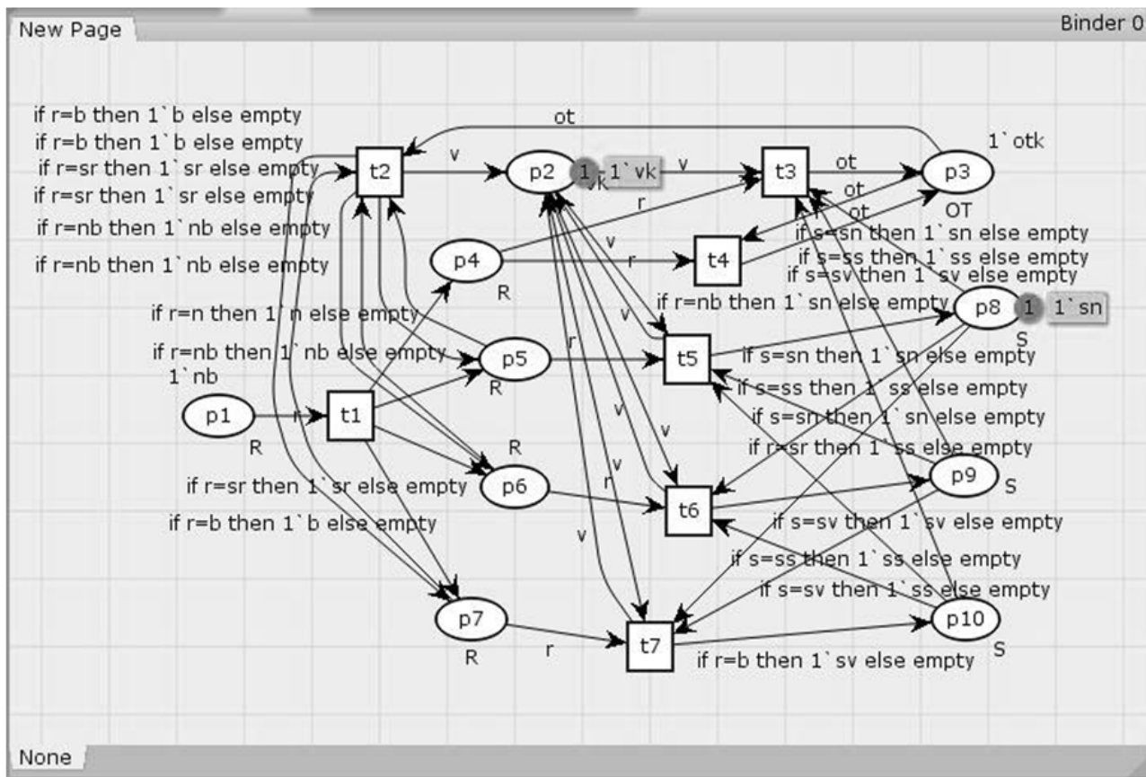
Рис. 4. Граф-модель нечеткой раскрашенной СП системы управления насосным агрегатом соответствующей 3-му шагу симуляции сети [Fig. 4. Graph model of the fuzzy colored PN control system of the pump unit corresponding to the 3-rd step of the network simulation]
