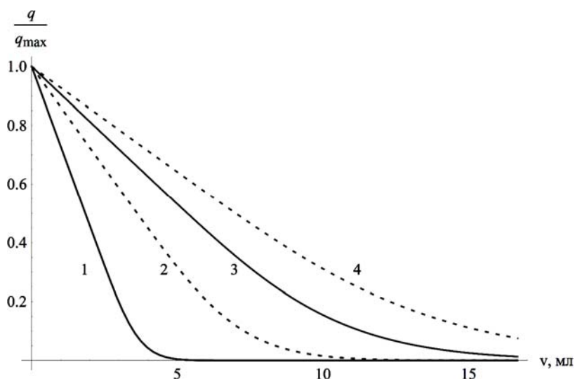
Рис. 2. Рассчитанная зависимость относительной остаточной емкости колонки от объема пропущенного «промывочного» раствора при различных величинах коэффициента распределения реагента.
