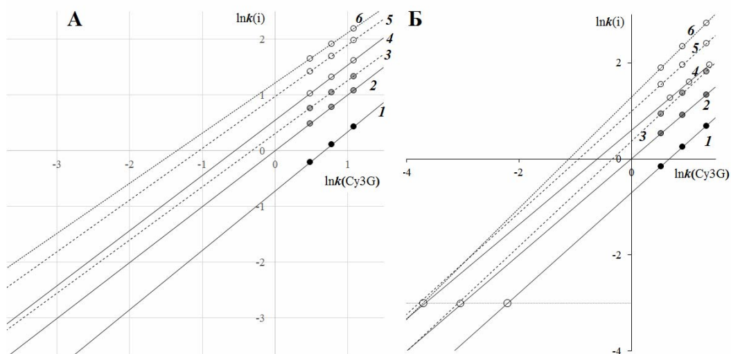
Рис. 1. Карта разделения 3-глюкозидов шести антоцианидинов А - колонка: 4.6×150 мм, MCI Gel CNP20/C04 (4 мкм); Б - колонка: 4.6×250 мм, Symmetry® C18, 5 мкм; элюенты системы «вода - ацетонитрил – 10 об.% муравьиной кислоты». 3-глюкозиды: 1 – дельфинидина (Dp3G); 2 - цианидина (Cy3G); 3 – петунидина (Pt3G); 4 – пеларгонидина (Pg3G); 5 – пеонидина (Pn3G); 6 – мальвидина (Mv3G).
