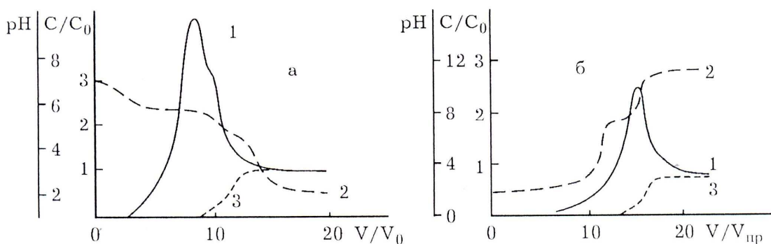
Рис. 2. Сорбция [10] тирозина (1) при pH = 2.0 анионитом АВ – 17 – 2П в ОН – форме (а) и катионитом КУ – 23 (30/100) (1') при pH = 9.0 (б). Изменение pH внешнего раствора (2, 2') и количества ионов Cl - (3) и ионов Na + (3'). C/C 0 – соотношение концентраций АК в элюате и в исходном растворе C 0 = 0.3 г/л. V/V 0 – отношение объема пропущенного раствора к объему слоя ионита.
