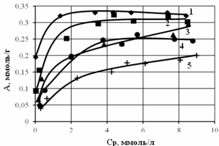
Рис. 1. Изотермы сорбции [\text{Cr}(\text{C}_2\text{O}_4)_3]^{3-} -ионов на свежесозданном феррогеле, полученном из хлорида железа (III) при \text{pH}_{\text{ос}} : 1 – 5,0; 2 – 6,0; 3 – 7,5; 4 – 8,0 и 5 – 9,0, в присутствии 0,5 М NaCl
