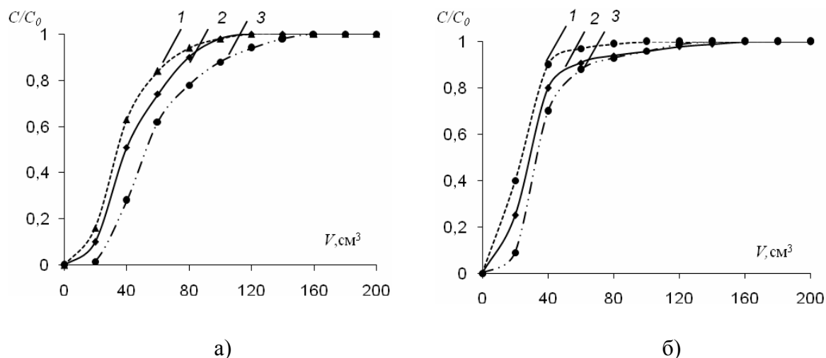
Рис. 3. Выходные кривые сорбции 0,01М раствора триптофана (а) и фенилаланина (б) анионообменником АН-251(Сl): 1 – 4 \text{cm}^3/\text{мин} ; 2 – 2 \text{cm}^3/\text{мин} ; 3 – 0,5 \text{cm}^3/\text{мин}
