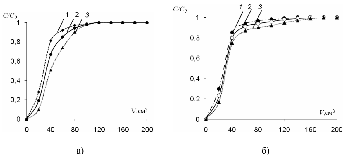
Рис. 1. Выходные кривые сорбции раствора триптофана (а) и фенилаланина (б) анионообменником АН-251(Сl) при различных концентрациях: 1 – 0,005 М; 2 – 0,01 М; 3 – 0,02 М (скорость пропускания 2 см 3 /мин).
