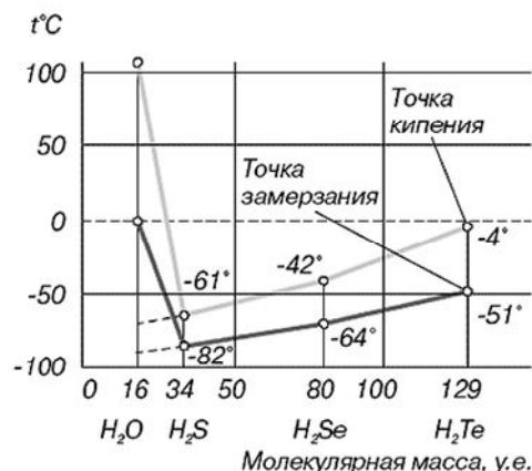
Рис. 2. Аномалия точек кипения и замерзания воды в сравнении с другими гидридами элементов с аналогичными химическими свойствами
