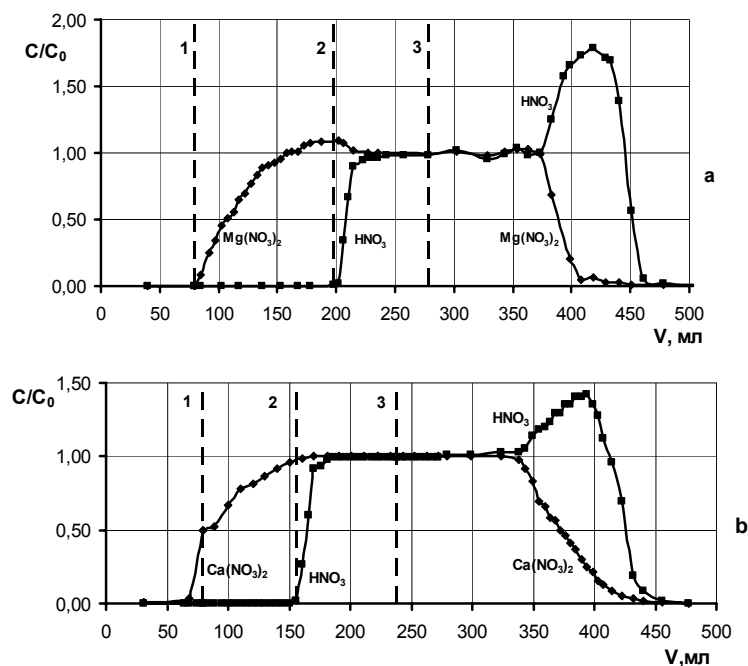
Рис.1. Выходные кривые сорбционного разделения компонентов из бинарных смесей: 1,33 М HNO_3 - 0,99 М Mg(NO_3)_2 (a) и 1,4 М HNO_3 - 0,95 М Ca(NO_3)_2 (b). Между прямыми (1) и (2) отмечены объемы фильтратов, выходящих из колонки после свободного объема и до появления кислоты. Слева от прямой (3) представлены кривые прямого фронтального анализа, справа - данные обратного фронтального анализа, полученные при десорбции кислоты водой
