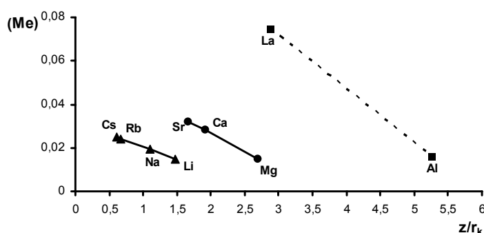
Рис.4. Величины сорбционной емкости сильноосновного анионита по нитратам различных металлов, достигаемые при пропускании через слой анионита в NO_3 -форме исходного раствора HNO_3 , содержащего 1 моль/л соответствующего нитрата, в зависимости от ионного радиуса и заряда катиона металла (в единицах: моль/л слоя на моль/л)
