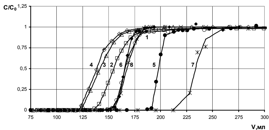
Рис. 2. Выходные кривые сорбции HNO_3 на анионите АВ-17 в NO_3^- - форме в присутствии нитратных солей, образованных различными катионами: 1- Li^+ , 2- Na^+ , 3- Rb^+ , 4- Cs^+ , 5- Mg^{2+} , 6- Sr^{2+} , 7- Al^{3+} , 8- La^{3+} . Участки выходных кривых, соответствующие вытеснению свободного объема колонки, на графиках не приведены.
