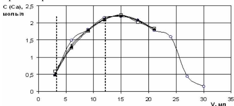
Рис. 6. Изменение концентрации нитрата кальция в ходе проведения повторяющихся циклических процессов сорбции-десорбции на колонке 1 с использованием натурального раствора минерализата костной ткани. Скорость пропускания раствора и воды - 0.5 мл/мин
