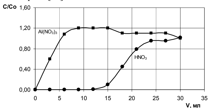
Рис. 3. Выходные кривые сорбции компонентов из модельного раствора 3 на колонке 1. Скорость пропускания раствора через колонку 0.5 мл/мин
