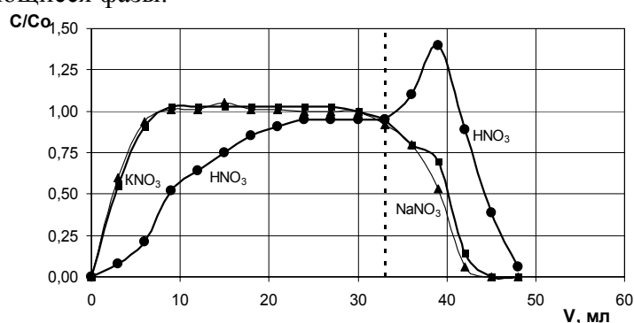
Рис. 1. Выходные кривые сорбции компонентов из модельного раствора 1 на колонке 1 и соответствующие кривые десорбции водой. Скорость пропускания раствора и воды через колонку 0,5 мл/мин. Пунктирная линия разделяет участки, соответствующие прямому и обратному фронтальному анализу
