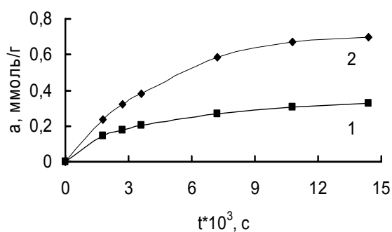
Рис. 1. Кинетические кривые адсорбции некаля анионитом ЭДЭ-10П в \text{OH}^- -форме при температуре 294 (1) и 308 (2) К
