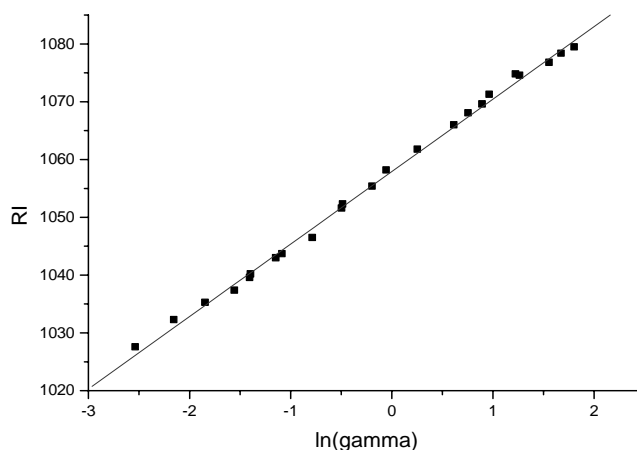
Рис. 1. Графическая иллюстрация линейности зависимости индексов удерживания ацетофенона от \ln\gamma для насадочной колонки с SE-30 (режим I) при температуре 70^\circ\text{C} . Параметры линейной регрессии (3): RI_{x,0} = 1057.9 \pm 0.2 , k = 12.5 \pm 0.1 , r = 0.998 , S_0 = 0.9
