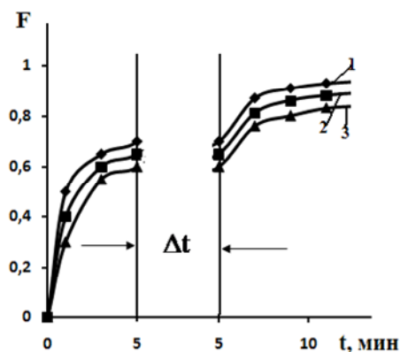
Рис. 1. Кинетические кривые сорбции ионов меди (1) бария (2) и иттрия (3) из 0,2 М азотнокислых растворов катионитом КБ-4п-2 при их совместном присутствии в опытах с прерыванием контакта фаз \Delta t=20 мин
