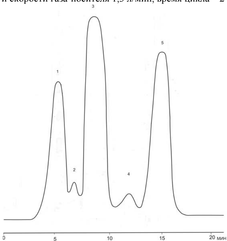
Рис. 4. Хроматограмма preparативного разделения метил-γ-трифторпропилсилоксанов.
