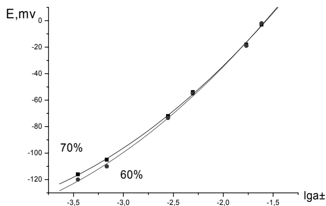
Рис. 7. Зависимость ЭДС гальванического элемента с мембраной от \lg a_{\pm} раствора \text{CaCl}_2 .
